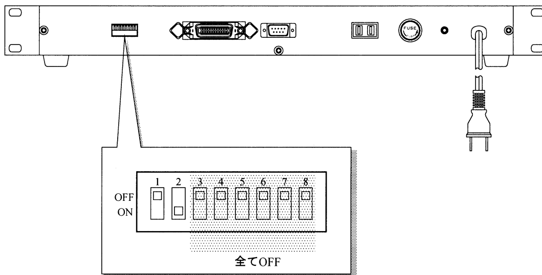
●ディップスイッチ拡大図
